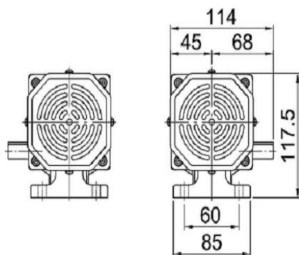
出力軸左方圖 LEFT SHAFT
